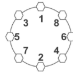
8-Lug Nuts
